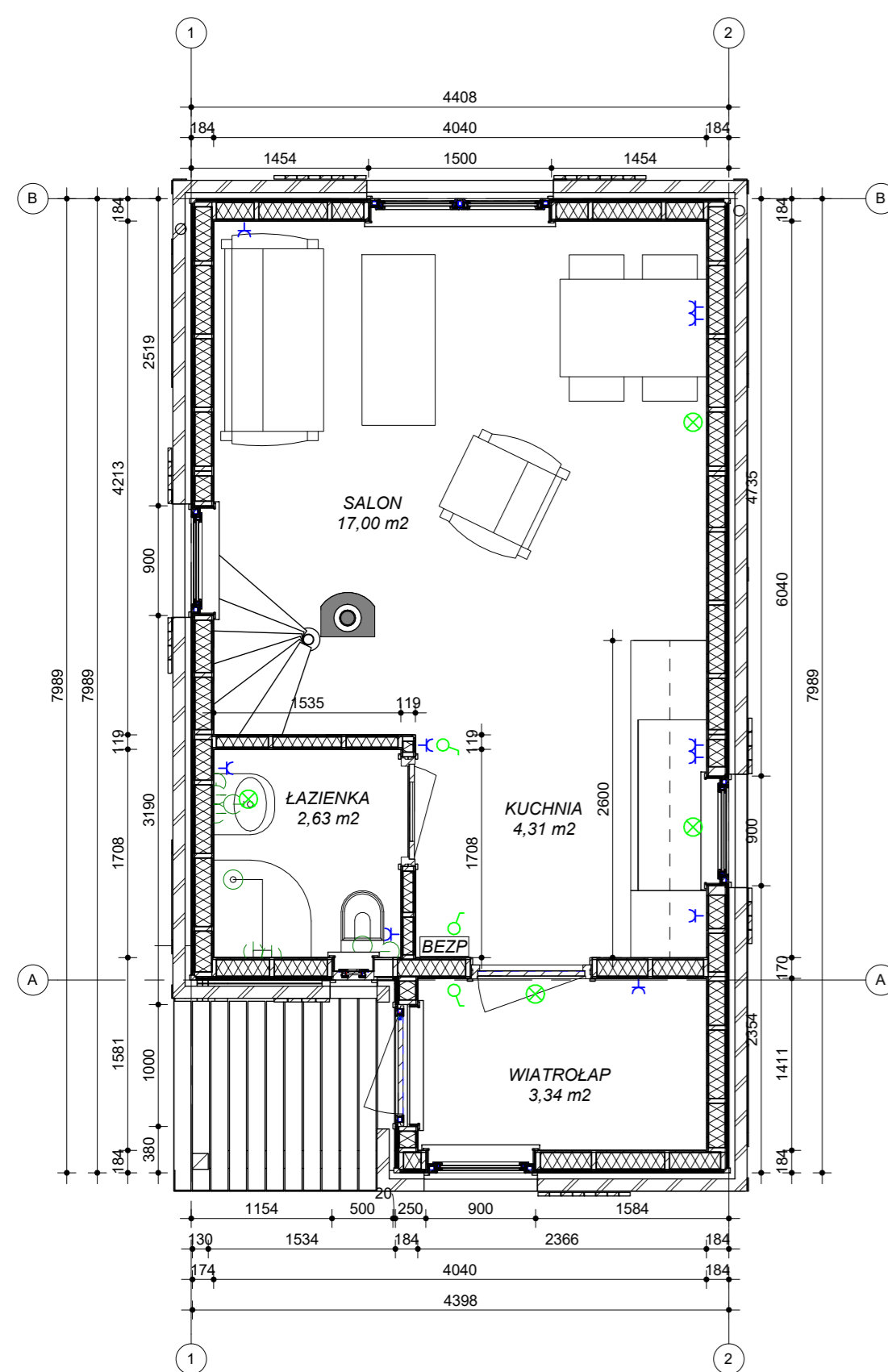
Rzut parteru
