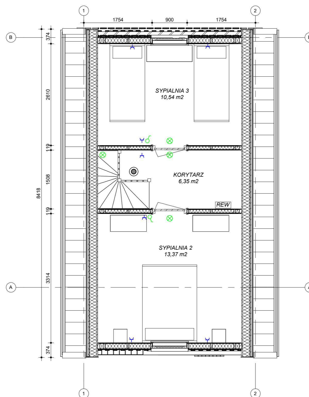
Rzut poddasza
